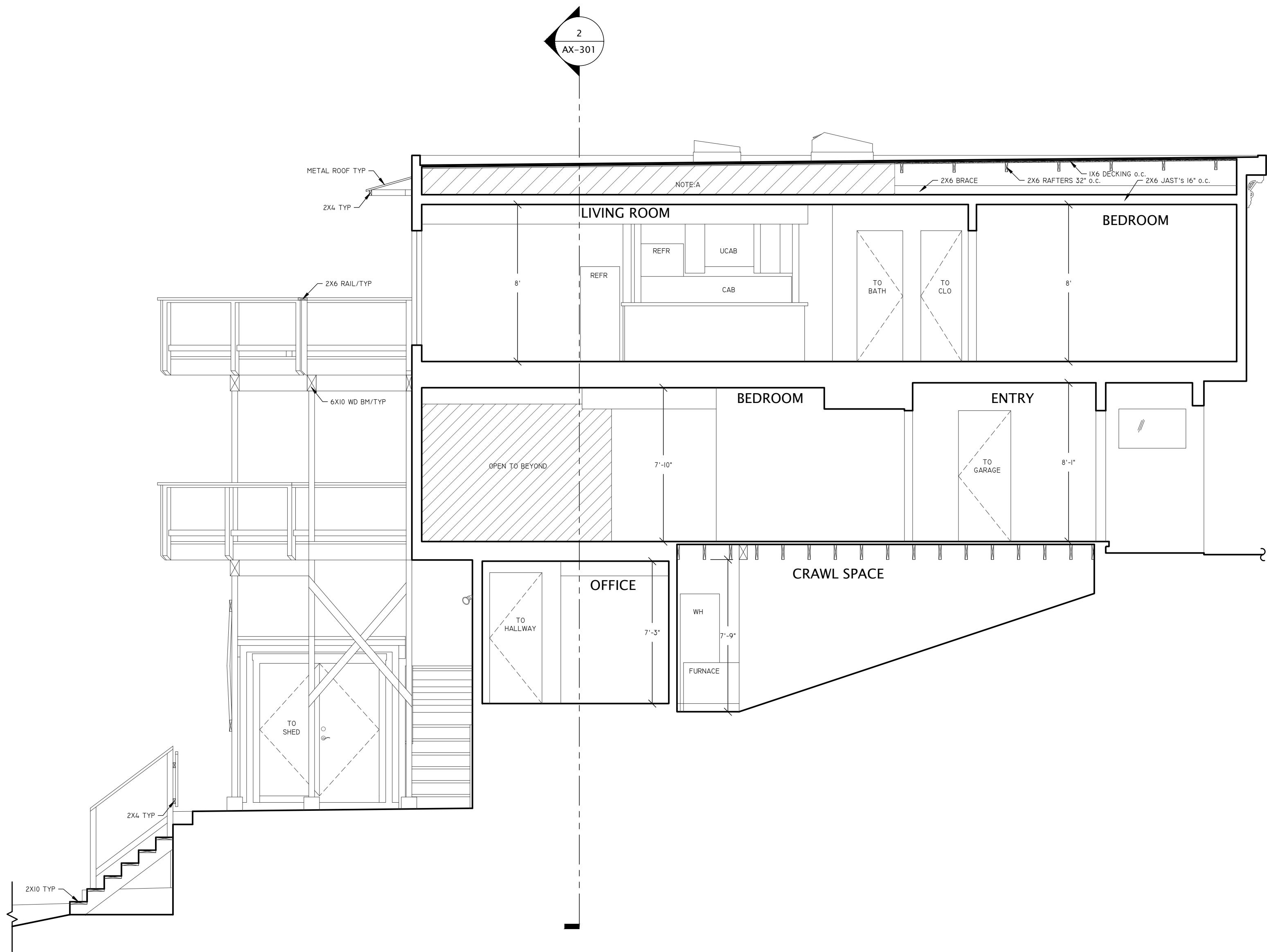
1 EXISTING LONGITUDINAL SECTION
